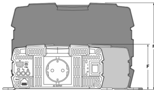
Bild 4. SP Serie Zeichnung (AC Ausgang/Vorderansicht)
